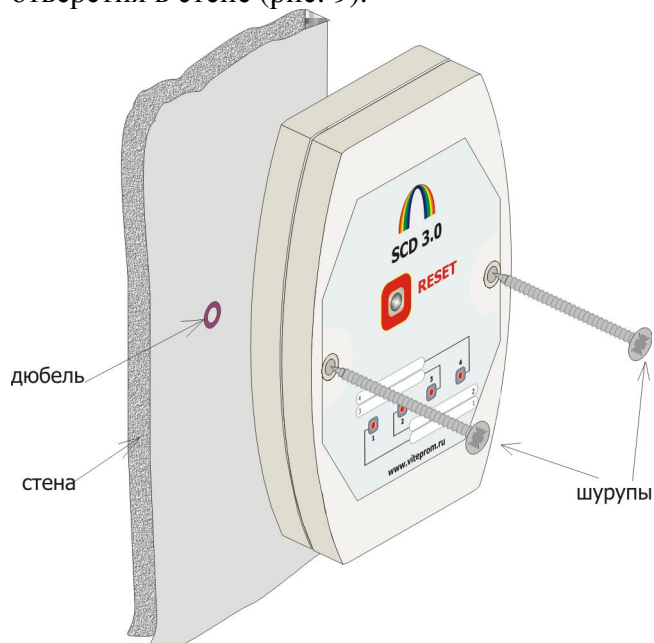
Рис.9 Монтаж блока SCD 3.0 на стену
