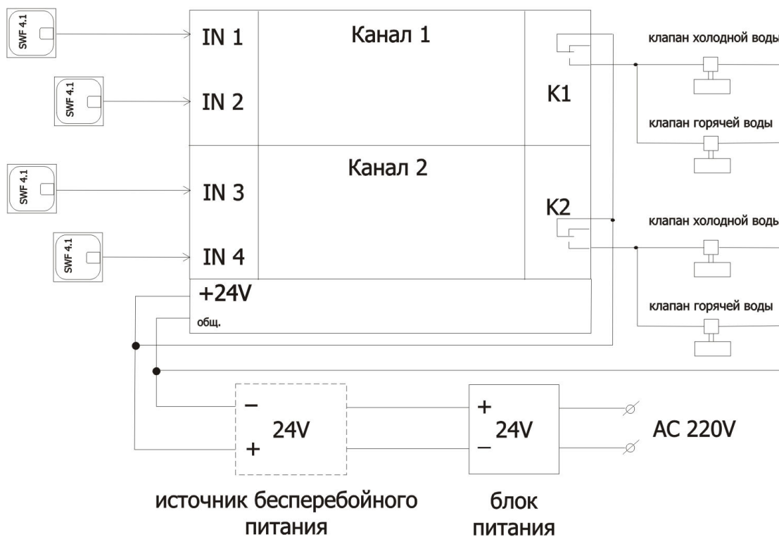
Рис.7 Схема включения блока управления для подключения 4 датчиков и 4 электромагнитных клапанов
