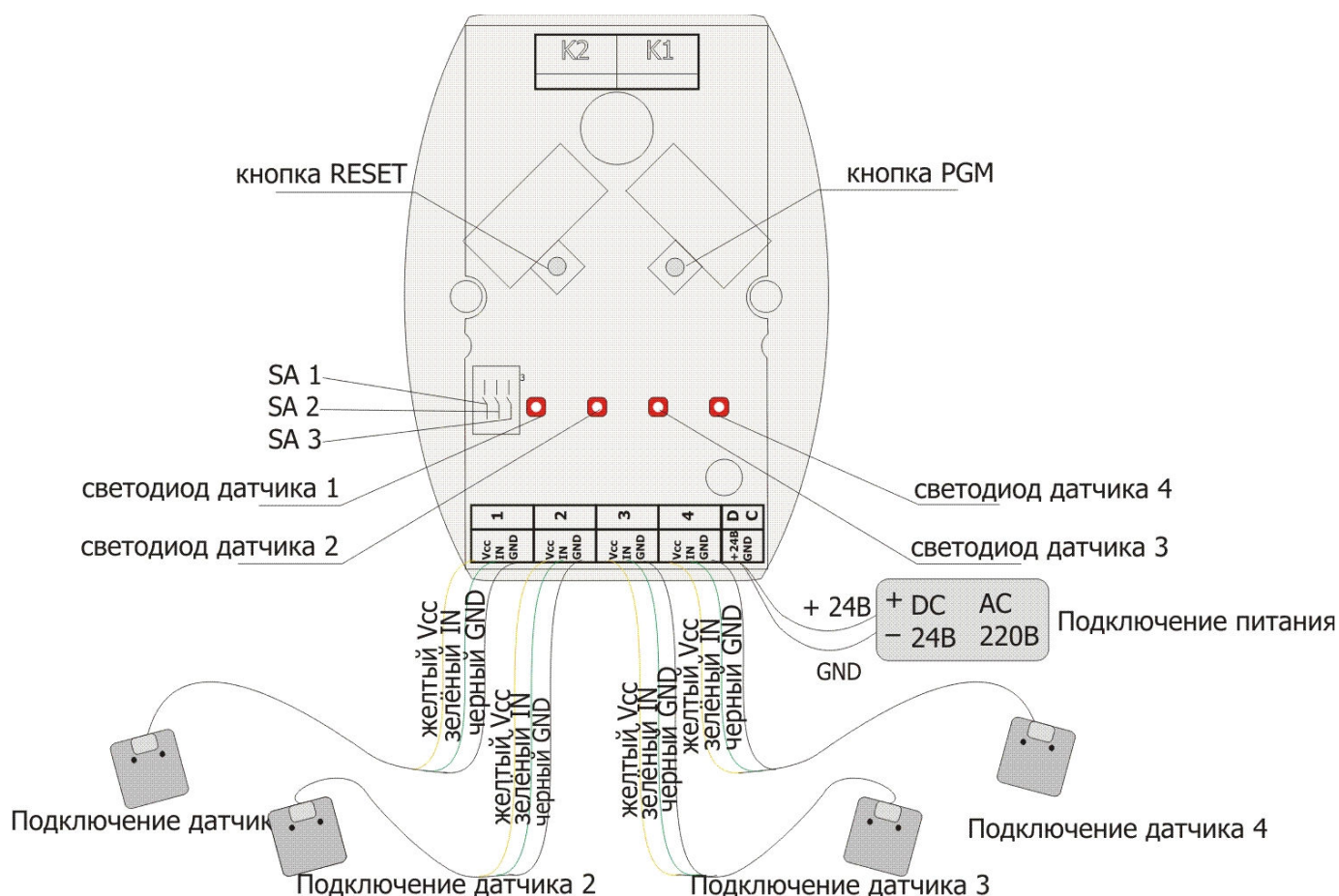
Рис.8 Схема подключения датчиков.
