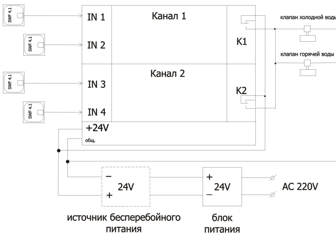
Рис.6 Схема включения блока управления для подключения 4 датчиков и 2 электромагнитных клапанов
