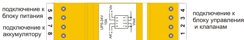
Рис 3. Источник резервного питания UPS-24V (вид сверху).
