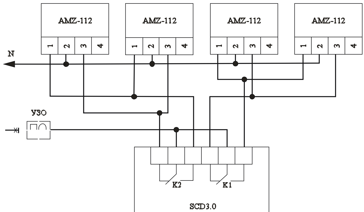
Рис.5. Подключение блока SCD3.0 к шаровым вентилям с электроприводами AMZ112
