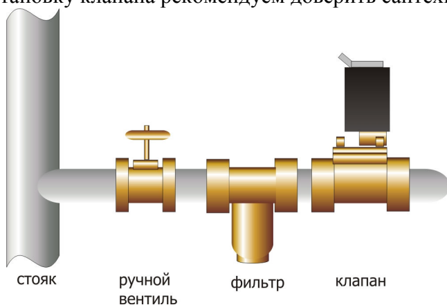
Рис 4. Установка клапана
